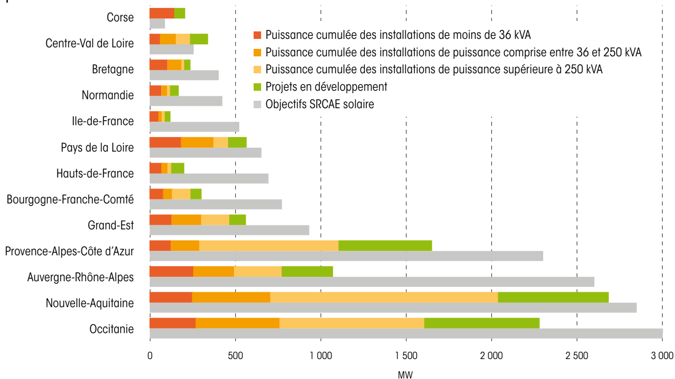
Puissances installées, projets en développement au 31 décembre 2017 et objectifs SRCAE pour le solaire
